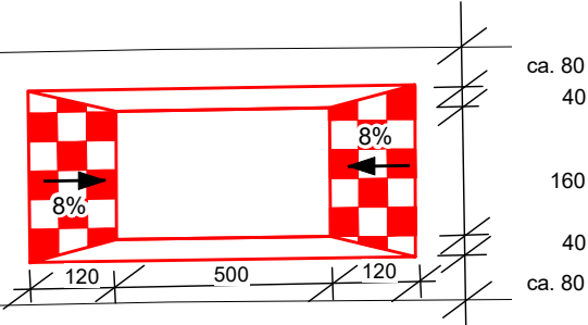
Detail: viereckförmiger Vertikalversatz ("Berliner Kissen")
